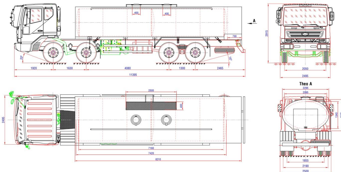
Xe chở sữa Daewoo M9AEF – 16m 3
