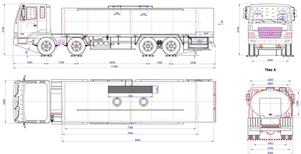
Xe chở sữa HYUNDAI HD310 – 16,5m 3
